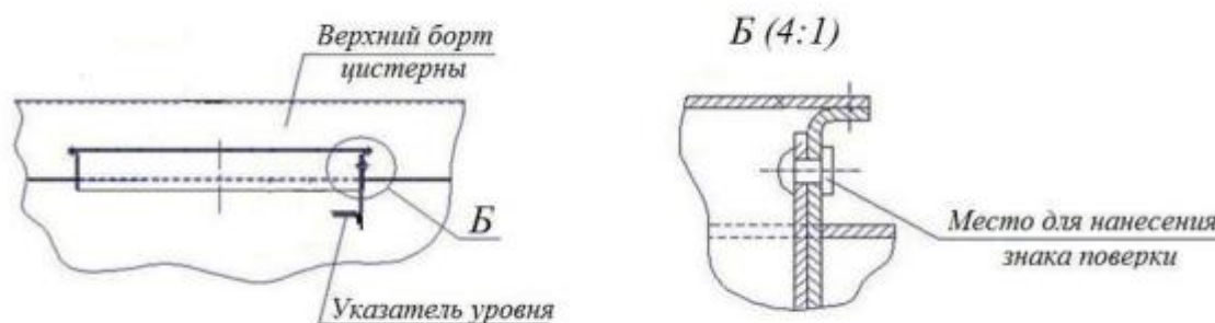
Рисунок 4 – Схема пломбировки от несанкционированного изменения положения уровня налива, обозначение места нанесения знака проверки
