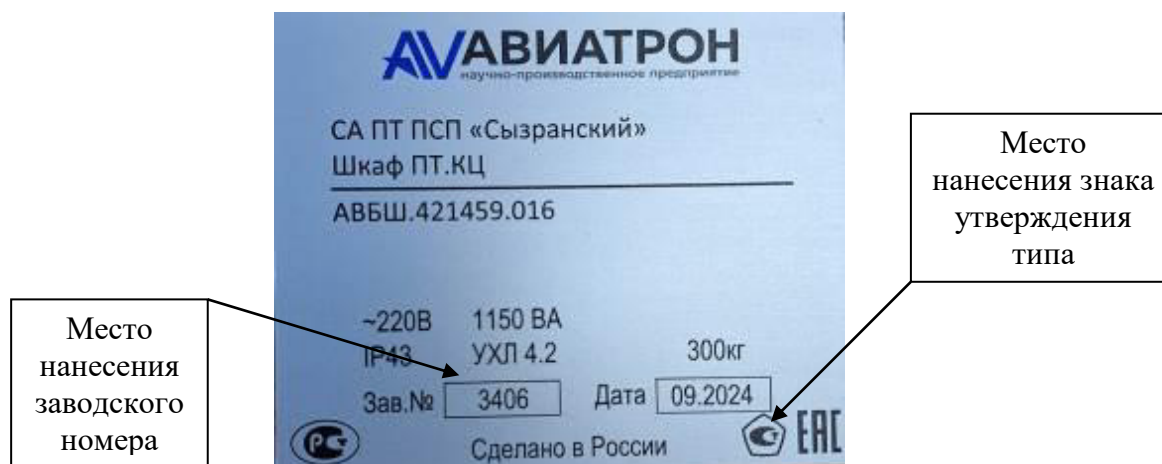
Рисунок 2 – Место нанесения знака утверждения типа и заводского номера
