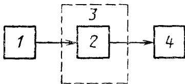
1—генератор ВЧ или СВЧ сигнала; 2—входной аттенюатор АС; 3—поверяемый АС, 4—установка для поверки аттенюаторов
