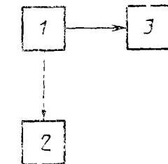
1—образцовая установка К2-38; 2—электронно-отсчетный частотомер; 3—поверяемый АС
