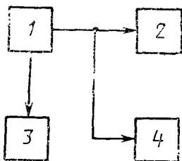
1—генератор гармонических сигналов; 2—поверяемый АС; 3—электронно-счетный частотомер; 4—измеритель уровня.
