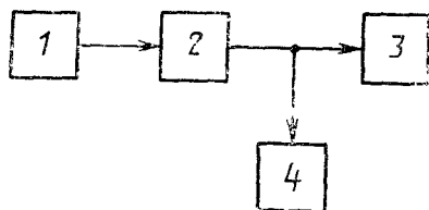
1—генератор ВЧ или СВЧ сигнала; 2—фильтр гармоник; 3—поверяемый АС; 4—образцовый измеритель уровня
