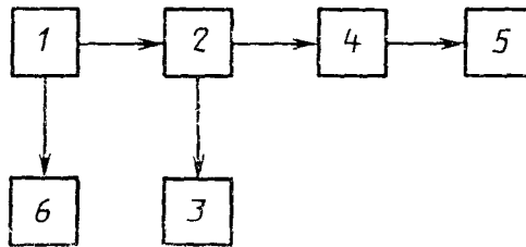
1—генератор ВЧ или СВЧ сигнала; 2—калибратор мощности; 3—мост постоянного тока; 4—согласующий аттенуатор; 5—поверяемый АС; 6—электронно-счетный частотомер
