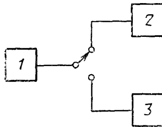
1—установка К2-34, 2—поверяемый АС, 3—модулометр
