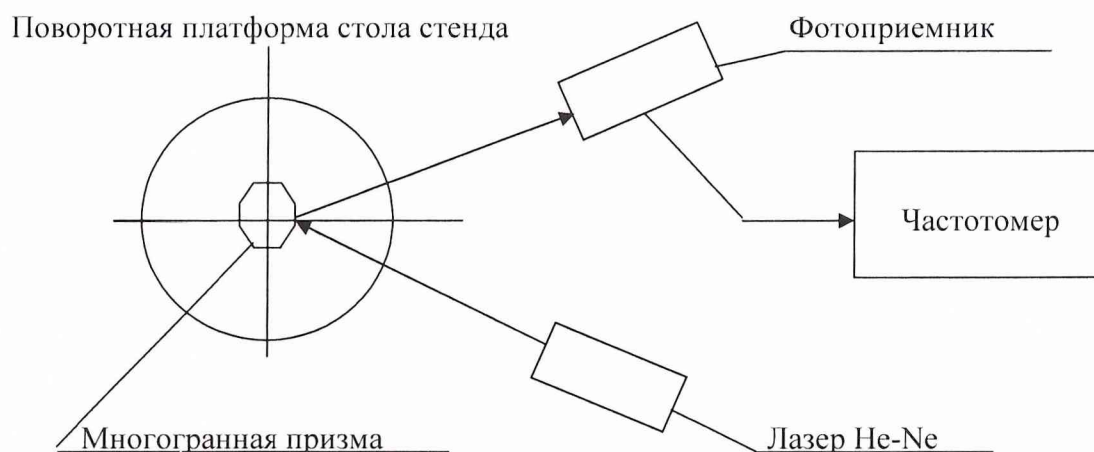
Рис.2 Схема измерений заданных значений угловой скорости платформы стола стенда
