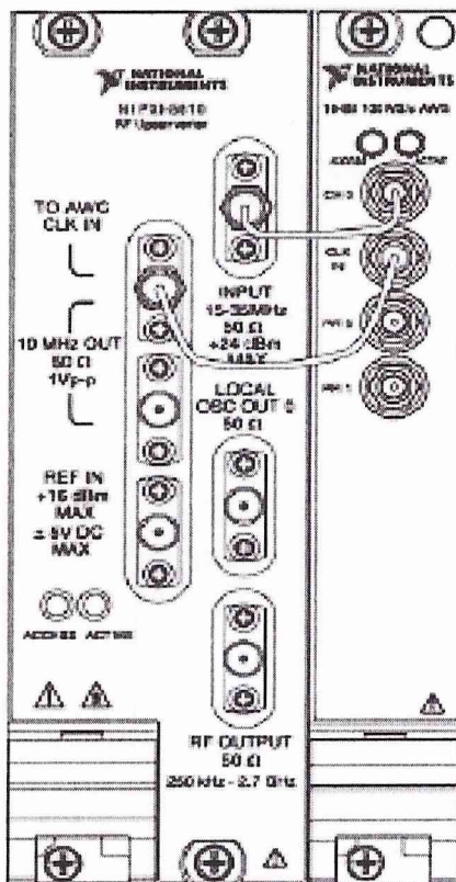
Рисунок 2 - Внешний вид передней панели генератора
