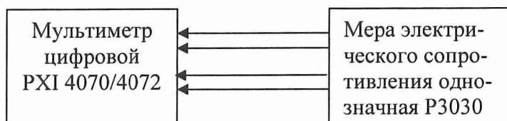
Рисунок 2. Структурная схема соединения приборов при номинальных значениях сопротивления от 100 Ом до 100 кОм
