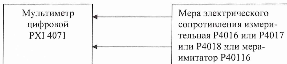
Рисунок 3. Структурная схема соединения приборов при номинальных значениях сопротивления от 1 МОм до 1 ГОм.
