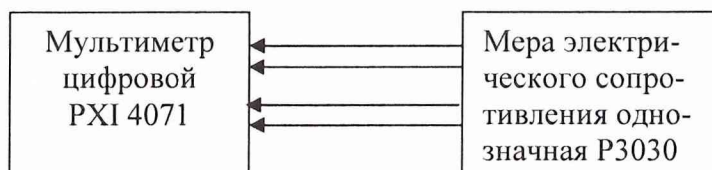
Рисунок 2. Структурная схема соединения приборов при номинальных значениях сопротивления от 10 Ом до 100 кОм
