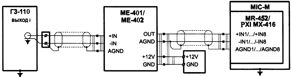
Рисунок 25 – Схема определения погрешности канала измерений частоты периодического сигнала: модуль MR-452 с нормализатором сигналов ME-401/ME-402, модуль PXI MX-416 с нормализатором сигналов ME-401/ME-402
