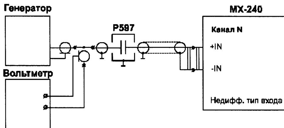
Рисунок 19 – Схема определения погрешности измерений электрического заряда модулей РХІ МХ-240 на диапазонах 1000, 10000.100000 пКл
