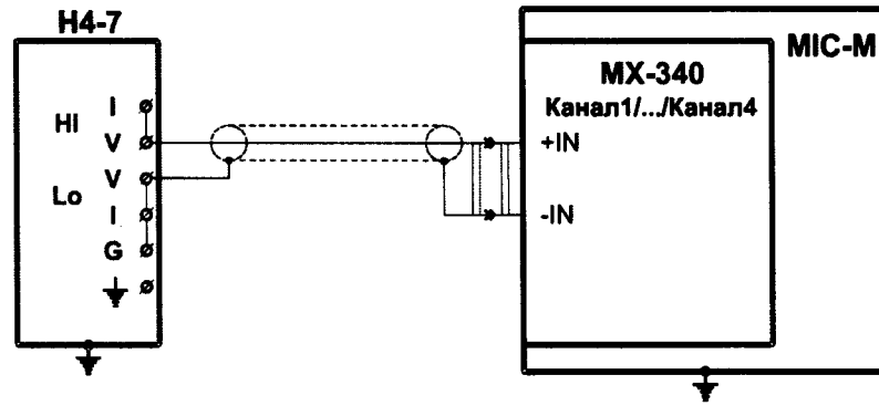
Рисунок 20- Схема определения погрешности измерений напряжения постоянного тока модуля PXI MX-340 в режиме недифференциальный вход
