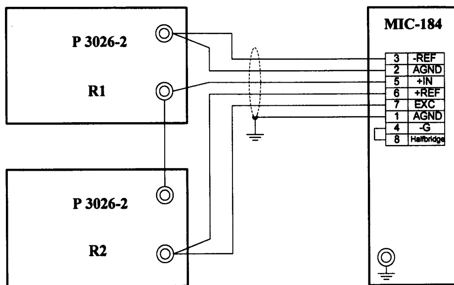
Рисунок 3 – Схема определения погрешности измерений относительного напряжения постоянного тока комплексов МІС-184
