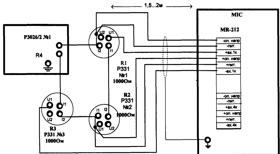
Рисунок 14 – Схема определения погрешности измерений относительного напряжения тензодатчиков модулей MR-212
