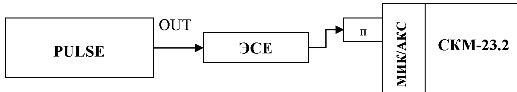
Рисунок 1 – Схема подключения
