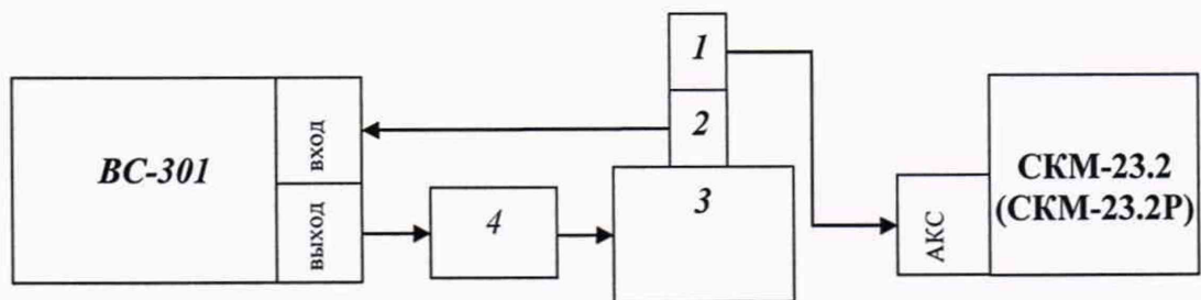
Рисунок 2 - Схема подключения
