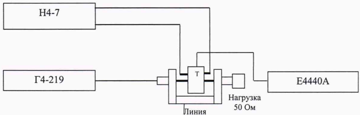
Рисунок 6 – Схема подключения
