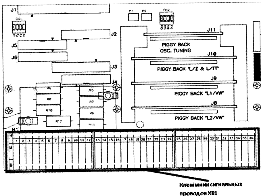
Рисунок 3 – расположение клеммника XB1 на «плате интерфейса машины» 3A4
