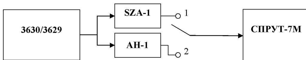
Рисунок 3 – Схема подключения
