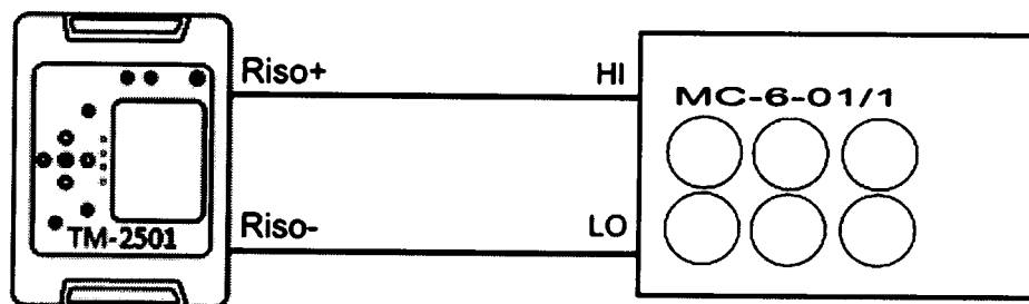
Рисунок 3 - Структурная схема определения абсолютной погрешности измерения сопротивления защитных проводников.
