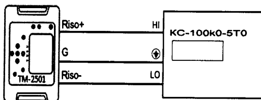
Рисунок 2 - Структурная схема определения абсолютной погрешности измерения сопротивления электроизоляции постоянным испытательным напряжением.
