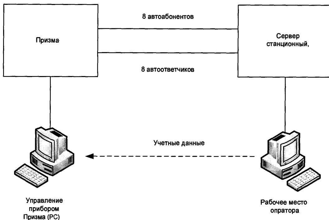
Рисунок 1. Схема поверки СИДС СС
