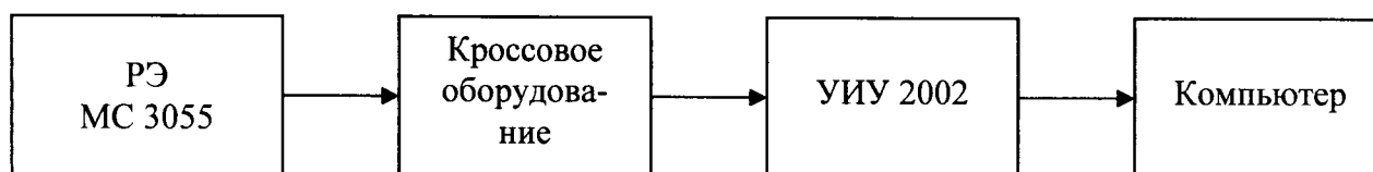
Рисунок 6 - Блок-схема поверки ИК сопротивления постоянному току, соответствующего значениям температуры, в диапазоне от 0 до 200 Ом
