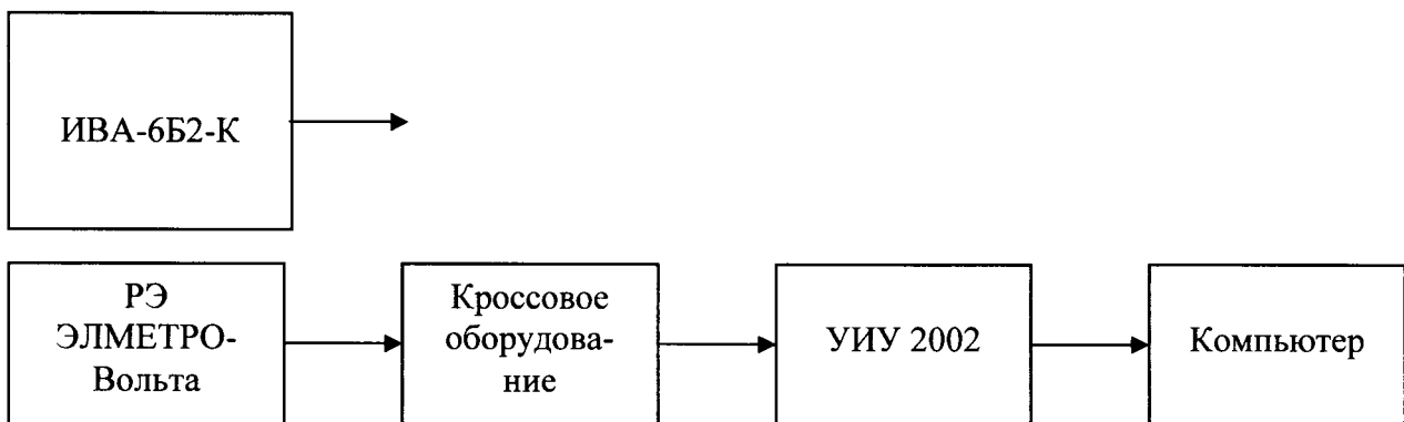
Рисунок 21 - Блок-схема поверки ИК относительной влажности атмосферного воздуха и ИК температуры датчиков влажности
