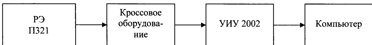
Рисунок 18 - Блок-схема поверки ИК силы постоянного тока, соответствующей значениям углового перемещения, в диапазоне от 4 до 20 мА
