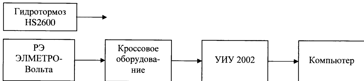
Рисунок 11 - Блок-схема поэлементной поверки ИК крутящего момента силы
