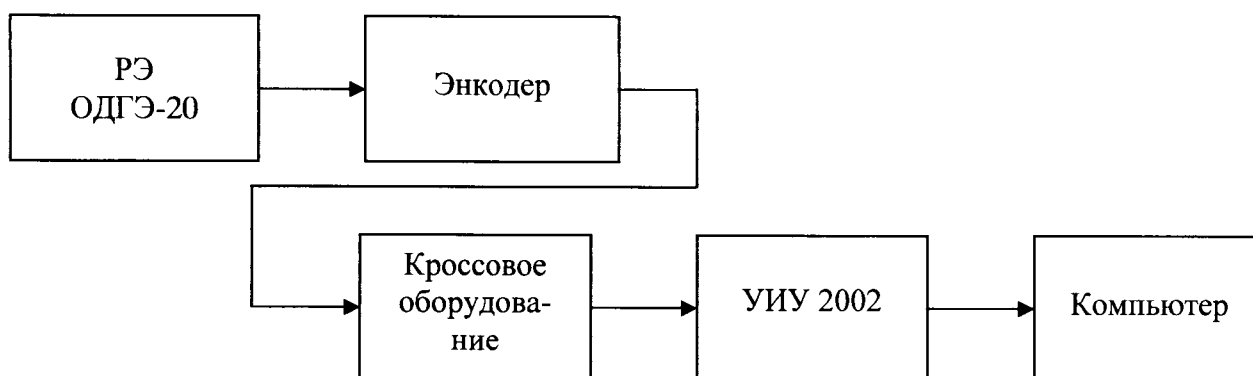
Рисунок 15 - Блок-схема комплектной поверки ИК угловых перемещений
