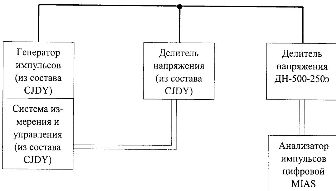
Рисунок 1 – Структурная схема проверки допускаемой относительной погрешности измерения и воспроизведения стандартизованных грозовых и коммутационных импульсов напряжения до 500 кВ
