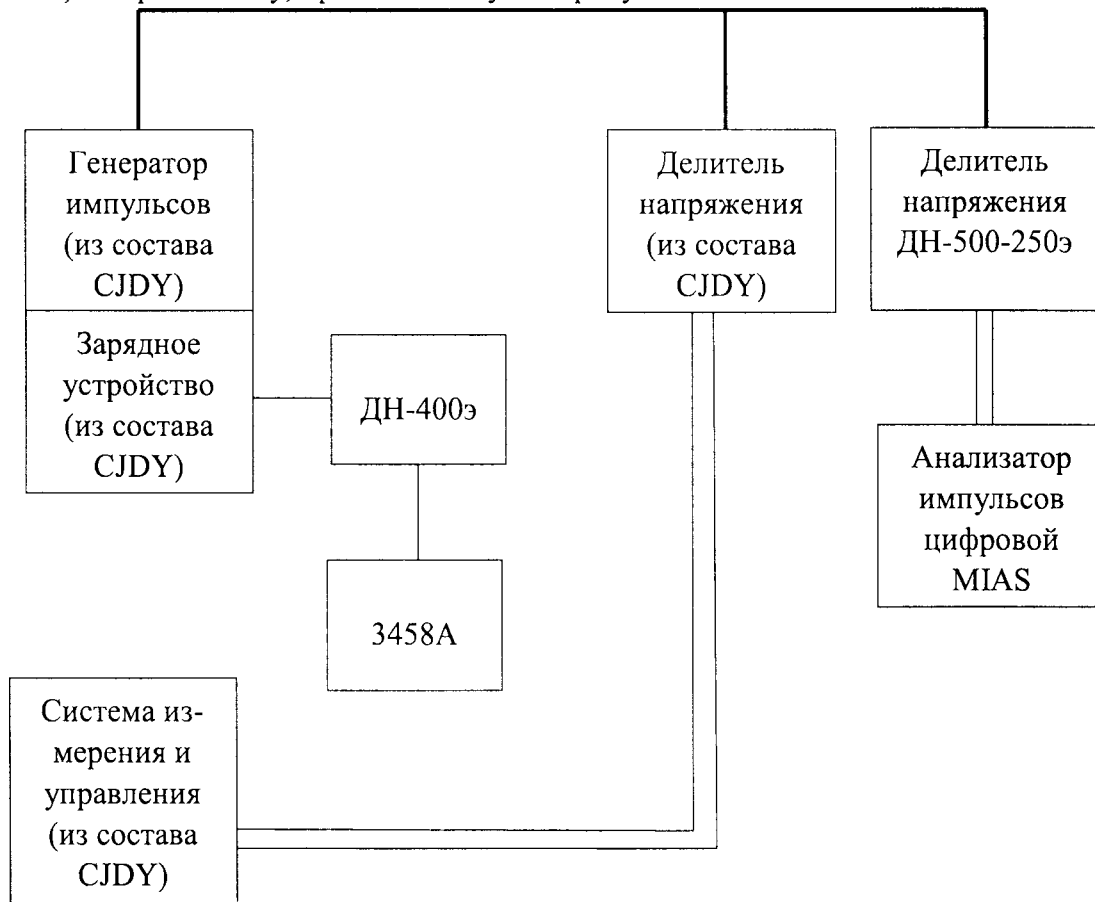
Рисунок 3 – Структурная схема проверки коэффициента полезного действия при воспроизведении стандартизованных грозовые (коммутационных) импульсов напряжения
