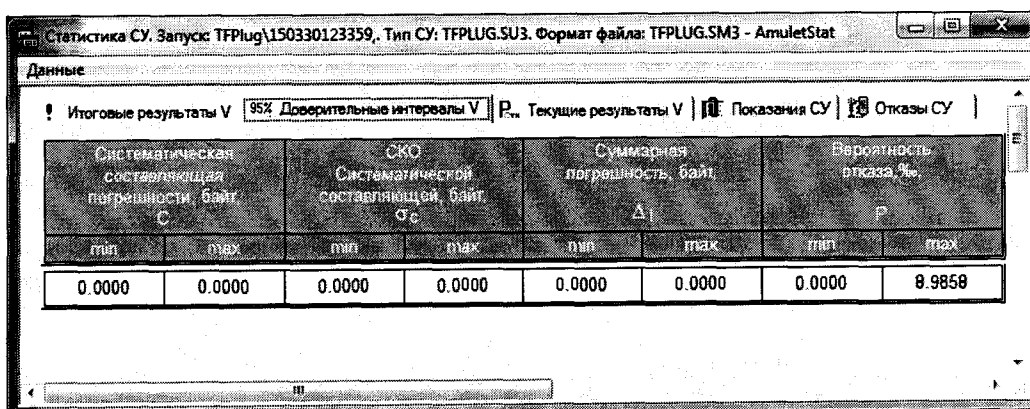
Рисунок 19 Доверительные интервалы
