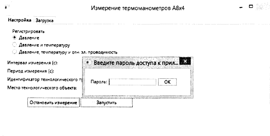
Рисунок 1 - Запуск программы
