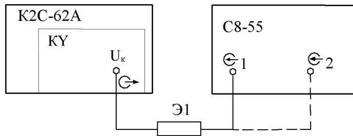
Рисунок 8.5 Схема соединения приборов для определения погрешности измерения напряжения между курсорами с делителем 1:10
