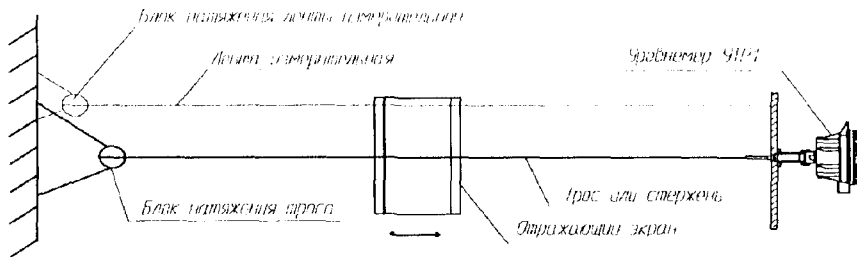
Рисунок 3. Схема измерения уровня (ВГП) датчиком УТР1 при помощи ленты измерительной (Вид сверху)
