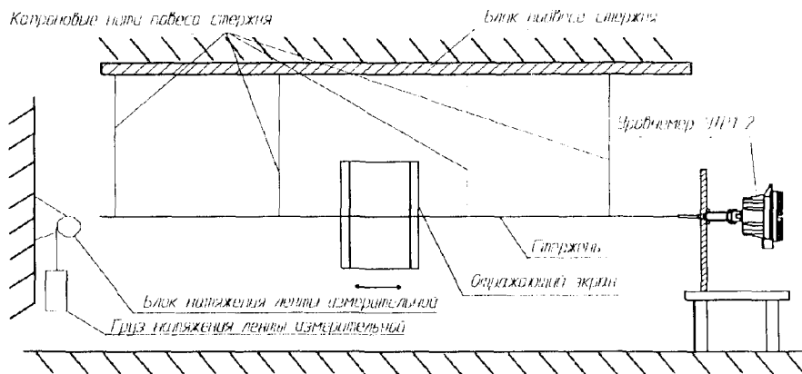
Рисунок 2. Схема измерения уровня (ВГП) датчиком УТР2 при помощи ленты измерительной (Вид сверху)
