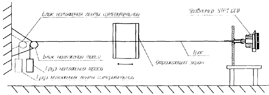
Рисунок 1. Схема измерений уровня (ВГП) датчиком УТР1 ВГП при помощи ленты измерительной (Вид сверху)
