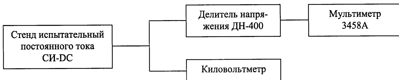
Рисунок 1 – Структурная схема проверки допускаемой основной относительной погрешности измерения напряжения постоянного тока
