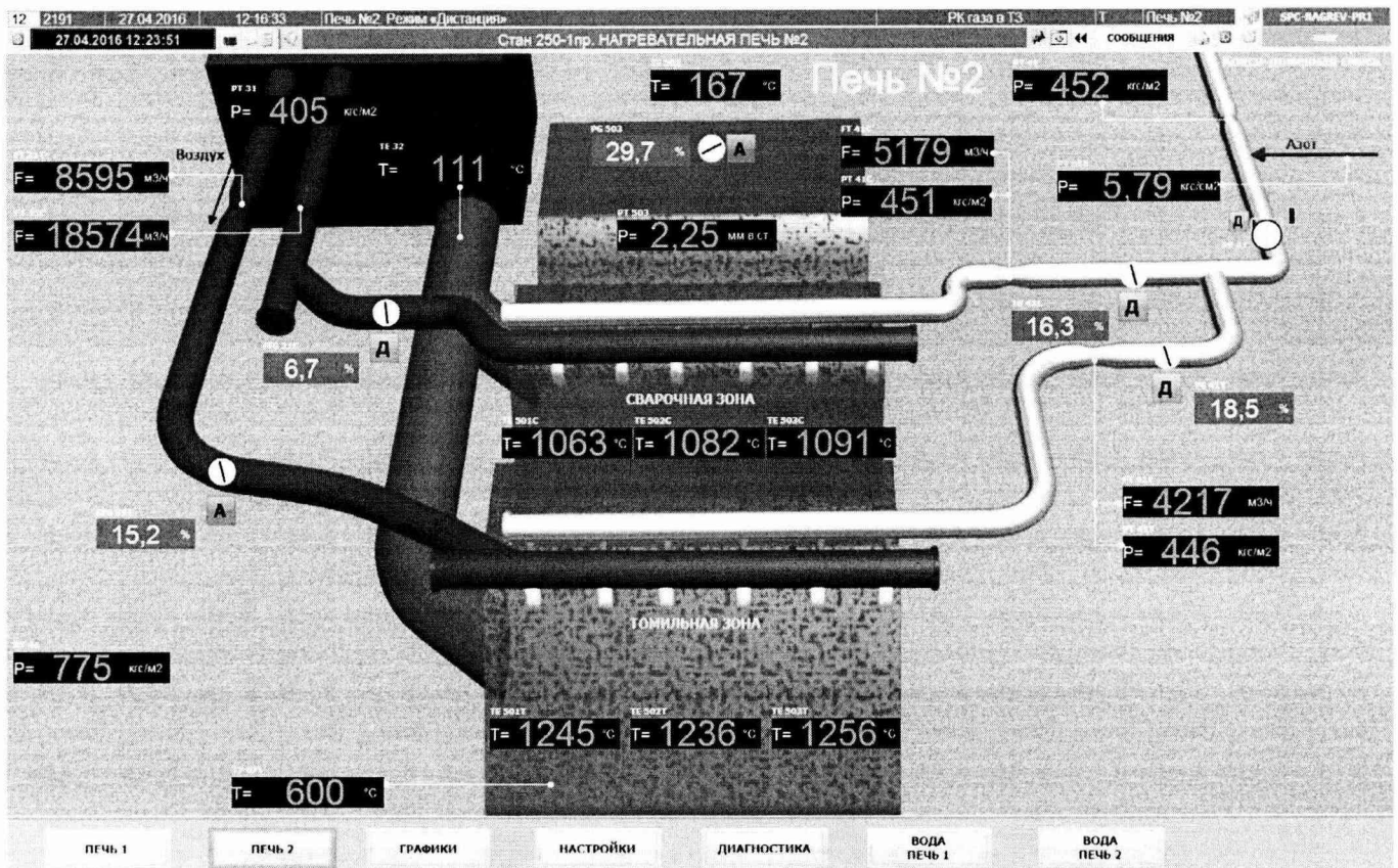
Рисунок 1 – Вид экранной формы «Печь № 2» программного обеспечения АРМ оператора
