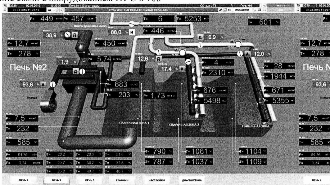
Рисунок 1 – Отображение значений технологических параметров на экранной форме «Стан 450. Нагревательная печь «№ 2»
