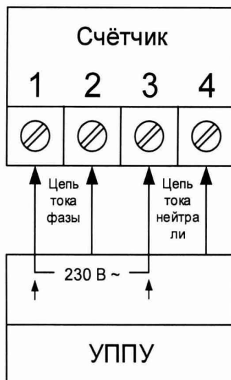
Рисунок А.1 - Подключение счётчика к УППУ
