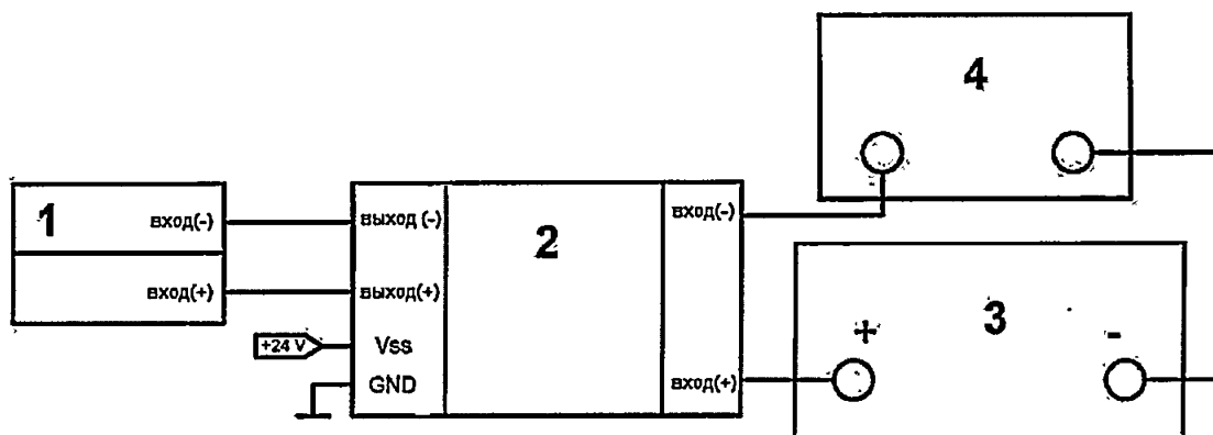
Рисунок А.3 – Схема соединения приборов при поверке входных аналоговых измерительных каналов типа 1 в составе с промежуточными измерительными преобразователями с гальванической развязкой (барьерами искробезопасности)
