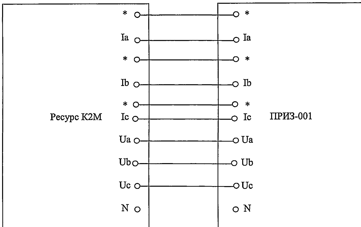
Рисунок 1 – Схема проверки допустимой основной приведенной погрешности измерения фазного напряжения, силы и частоты переменного тока
