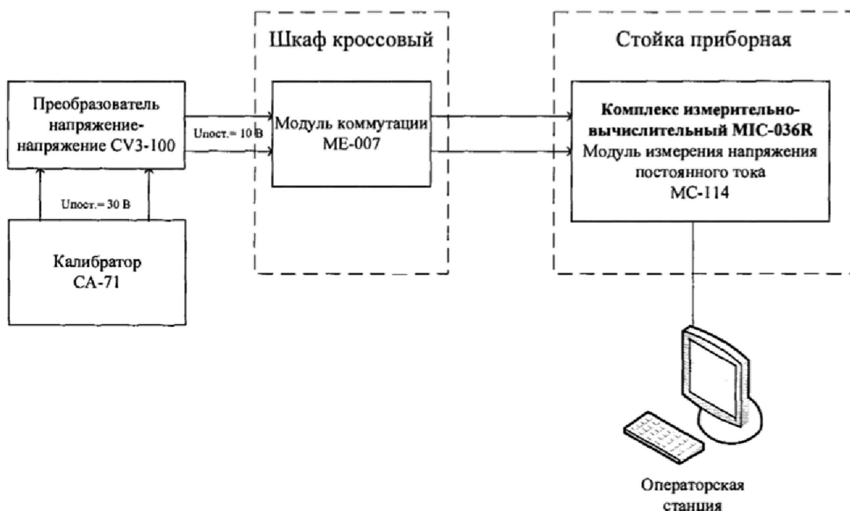
Рисунок 22 - Схема поверки ИК напряжения постоянного тока
