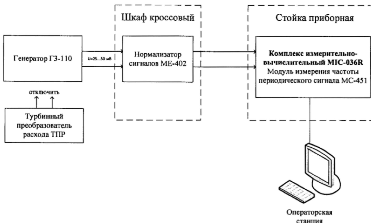
Рисунок 12 – Схема поверки ИК расхода (прокачки) рабочей жидкости и масла
