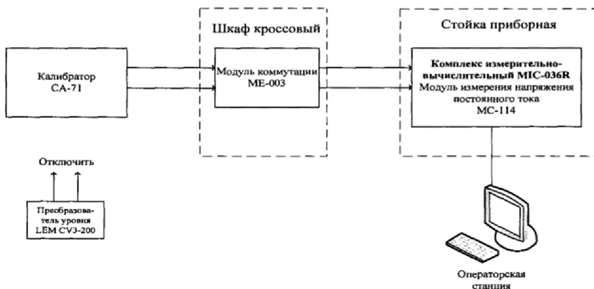
Рисунок 19 - Схема поверки ИК напряжения переменного тока
