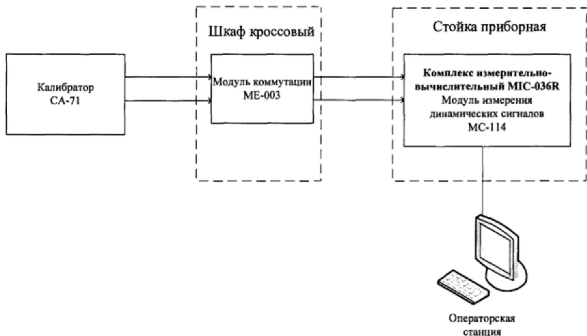
Рисунок 16 - Схема поверки ИК напряжения постоянного тока
