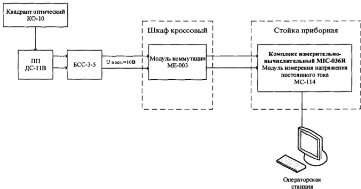
Рисунок 17 - Схема поверки ИК угловых положений РУД и створок реактивного сопла с ПП сельсинного типа
