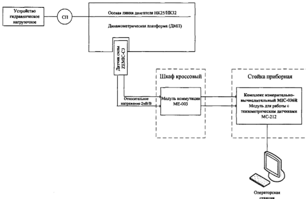
Рисунок 18 – Схема поверки ИК силы от тяги
