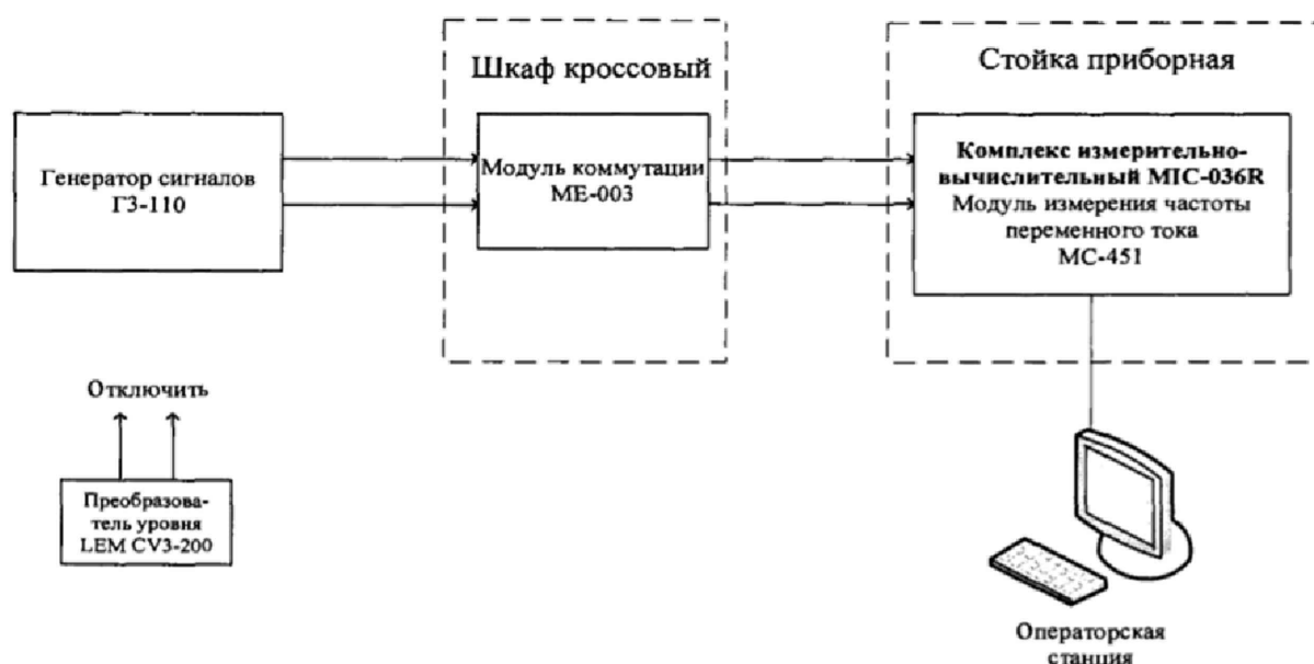
Рисунок 20 - Схема поверки ИК частоты переменного тока
