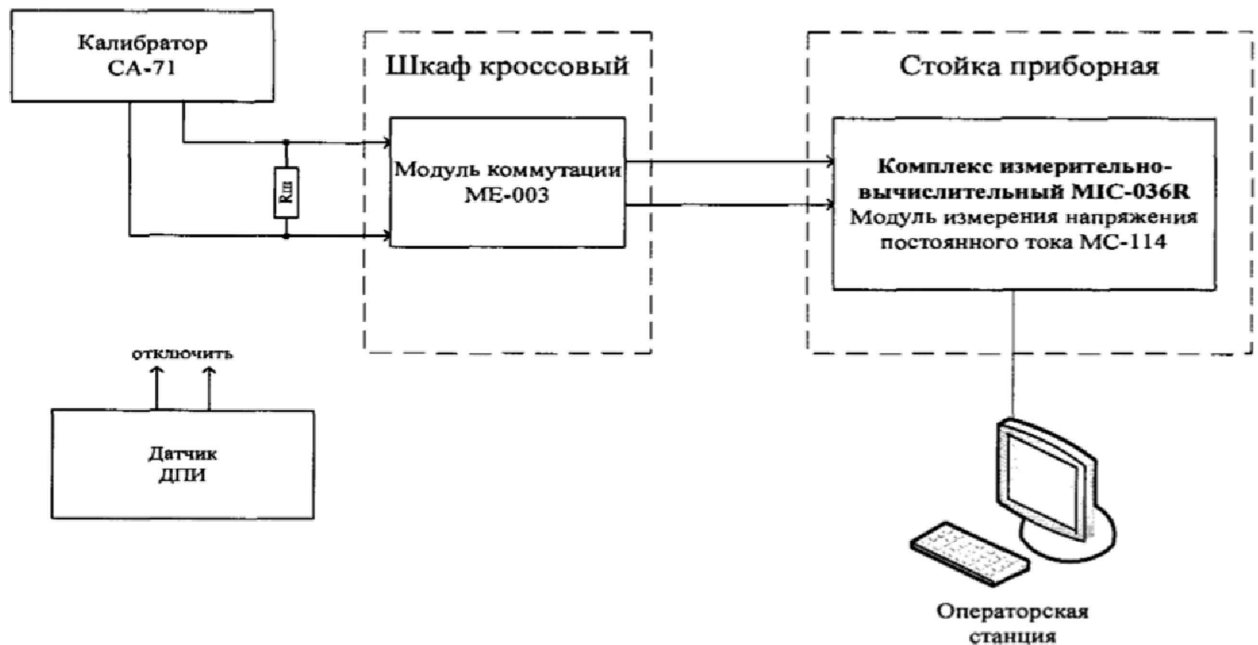
Рисунок 24 – Схема поверки ИК тока датчиков ДПИ
