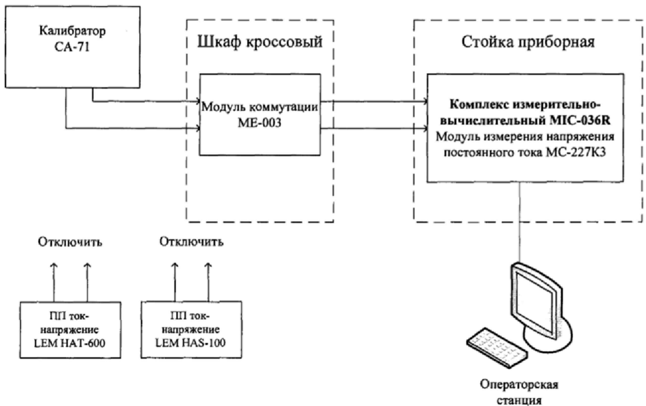
Рисунок 23 - Схема поверки электрической части ИК силы постоянного тока
