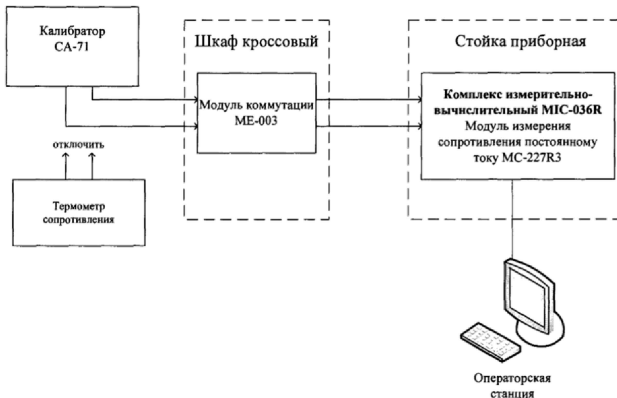
Рисунок 15 - Схема поверки ИК температуры жидких и газообразных сред с ПП терморезистивного типа (термометрами сопротивления)
