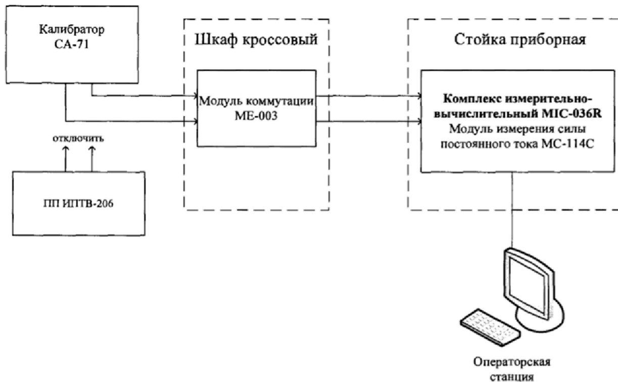
Рисунок 25 – Схема поверки ИК температуры и влажности атмосферного воздуха
