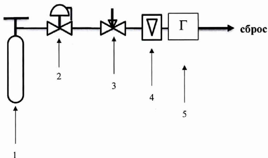
1 - Баллон с ПГС; 2 - Регулятор давления (редуктор); 3 - регулировочный вентиль; 4 – ротаметр; 5 – газоанализатор.
