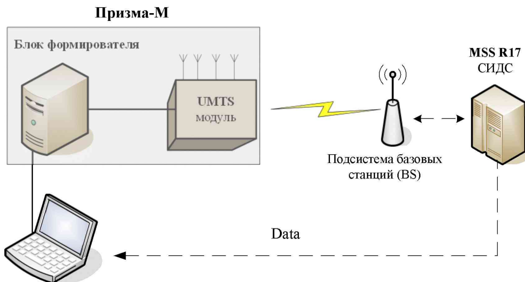
Рисунок 2 - Схема поверки СИДС по радиотракту
