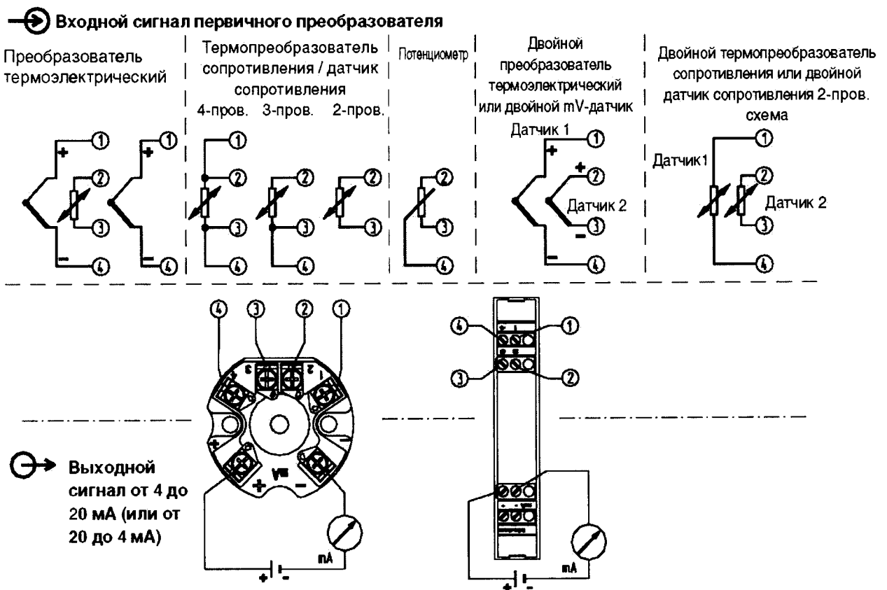
Рисунок 1 – Схема подключения T32.1S, T32.3S
