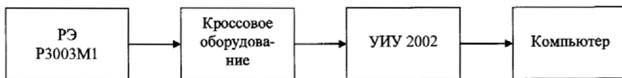
Рисунок 8 - Блок-схема поверки ИК напряжения постоянного тока, соответствующего значениям температуры
