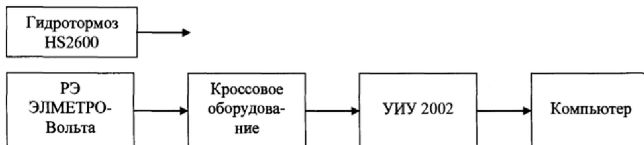
Рисунок 11 - Блок-схема поэтапной поверки ИК крутящего момента силы
