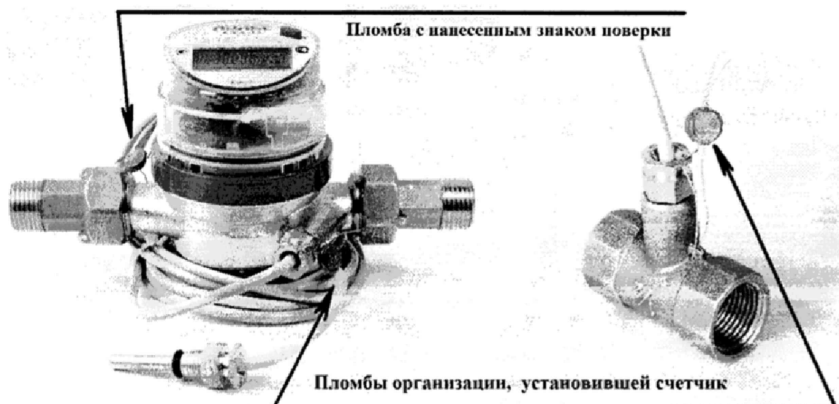
Рисунок 3 – Схема пломбировки теплосчетчиков
