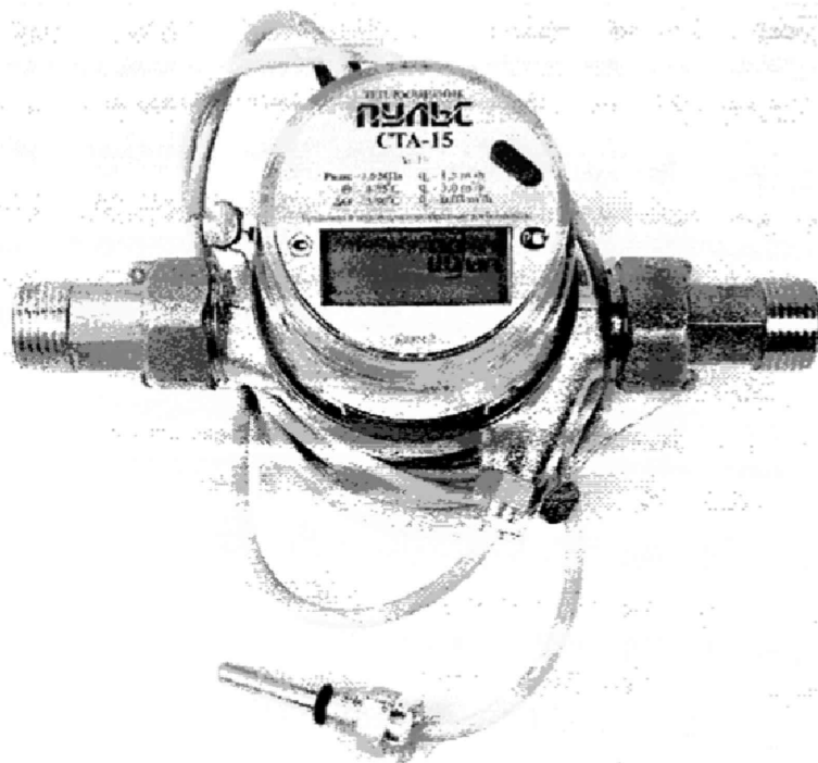
Рисунок 1. Внешний вид теплосчетчика.
