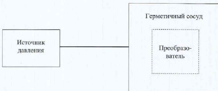
Рисунок 1 – Структурная схема проверки герметичности системы
