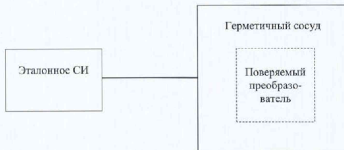
а) Схема определения приведенной (к диапазону измерений) погрешности измерений абсолютного и гидростатического давлений для преобразователей без оптического считывателя USB
