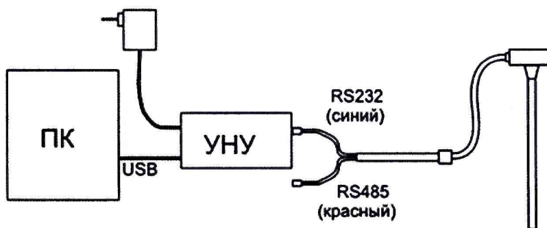
Рисунок А.3 – Схема подключения LLS 30160к ПК по интерфейсу RS-232
