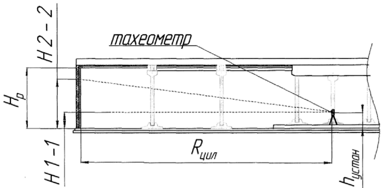
Рисунок А.3 – Схема измерений диаметра резервуара
