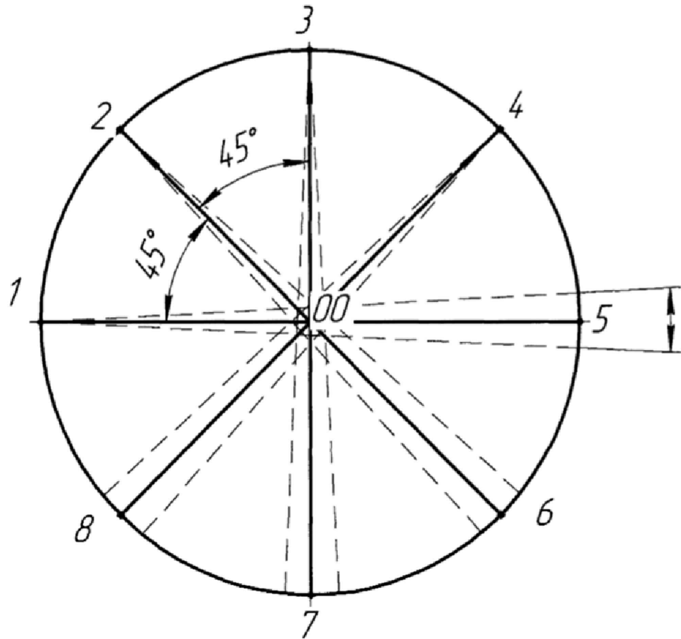
Рисунок А.2 – Схема определения центра днища резервуара
