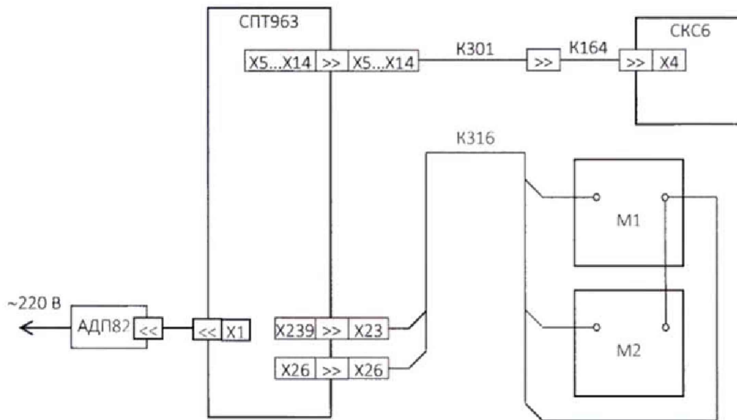
Рисунок 11.2 – Схема проверки. M1, M2 – магазин сопротивлений P4831
