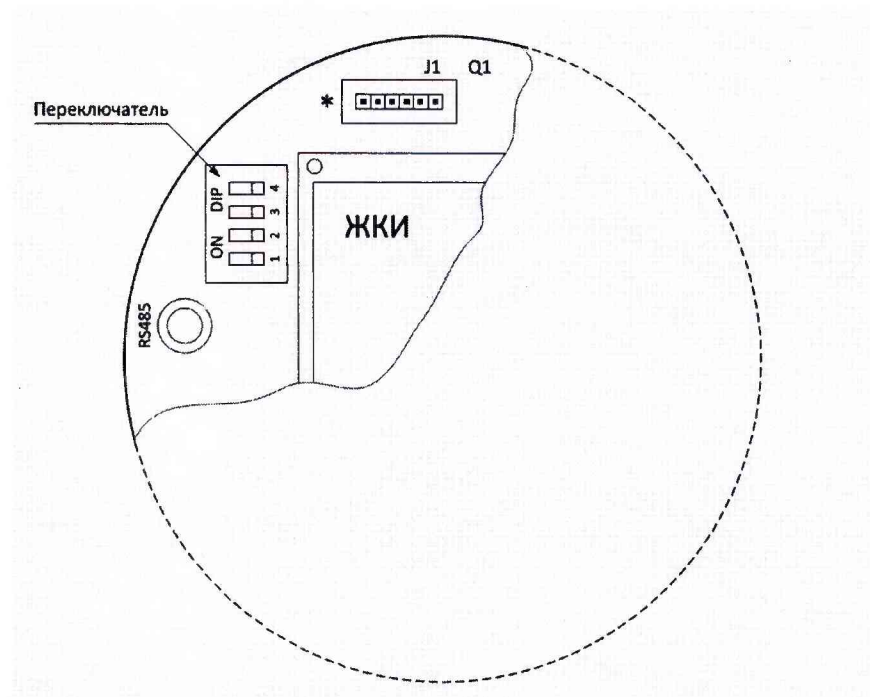
Рисунок А.1 – Схема расположения переключателя на печатной плате электронного блока расходомера-счетчика
