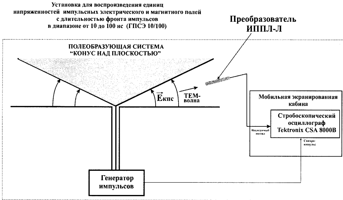
Рисунок 3 – Схема исследований при определении характеристик ИППЛ-Л
