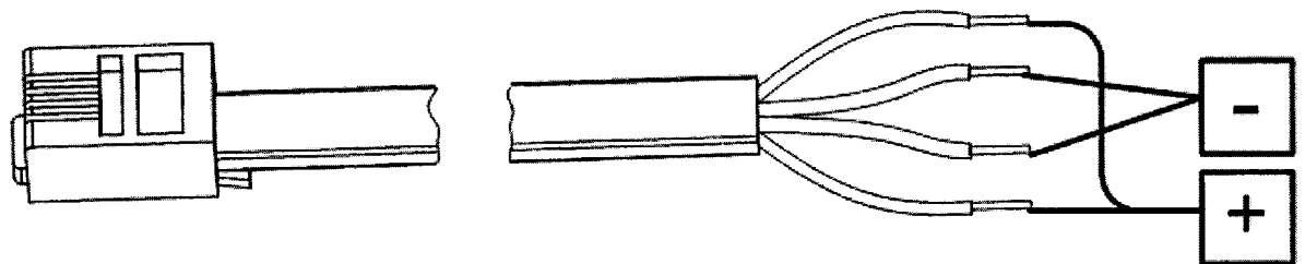
Рисунок 8 Подключение расходомеров
