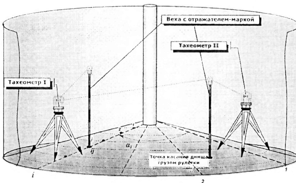
Рисунок А.6 Определение параметров днища резервуара при наличии в резервуаре центральной трубы
