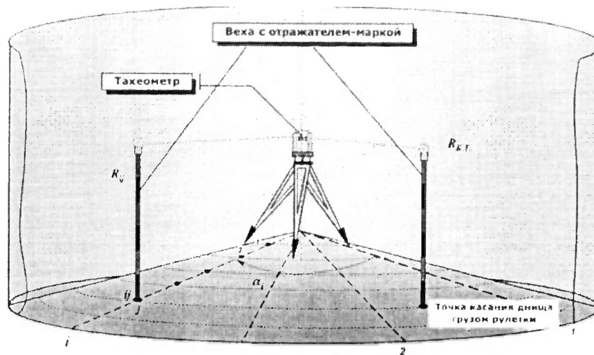
Рисунок А.5 Определение параметров днища резервуара
