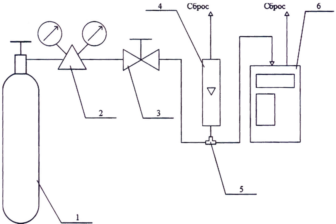
1 – источник ГС; 2 – редуктор баллонный; 3 – вентиль точной регулировки трассовой; 4 – ротаметр (индикатор расхода); 5 – тройник; 6 - газоанализатор (показан условно)
