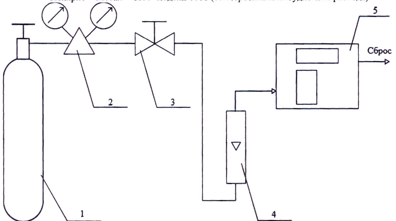
Рисунок 1 – Схема (рекомендуемая) подачи ГС из баллонов под давлением на газоанализаторы "Полярис" "Метан – CH 4 " модели 1001 (со встроенным побудителем расхода)
