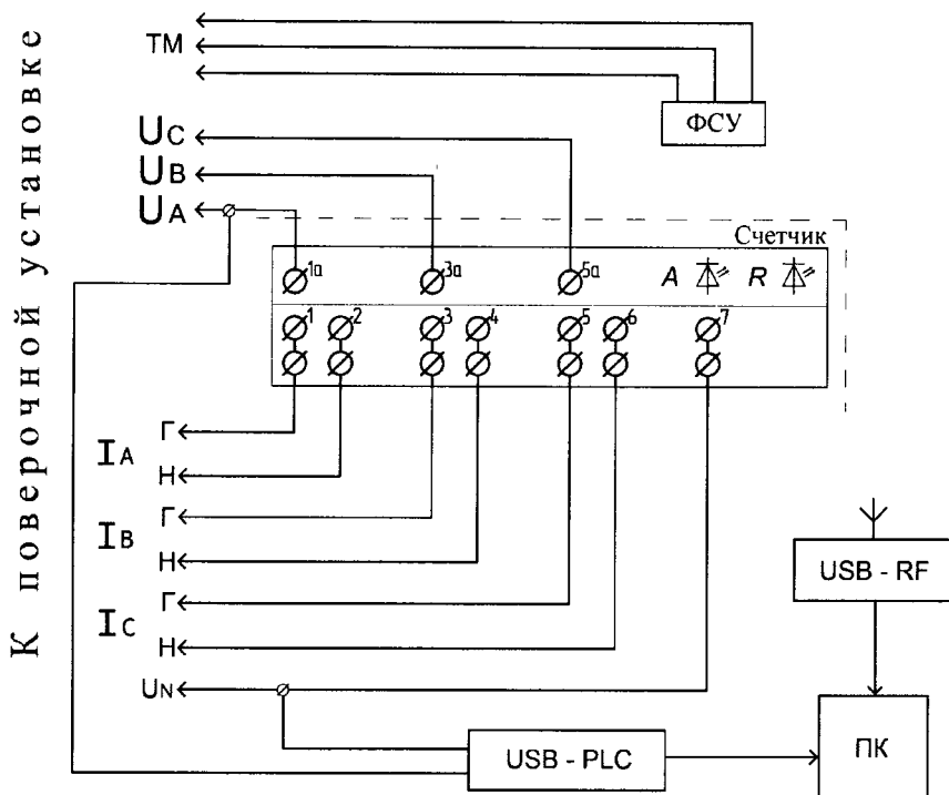
Рисунок Б.1 – Схема включения счетчиков РиМ 489.1Х
