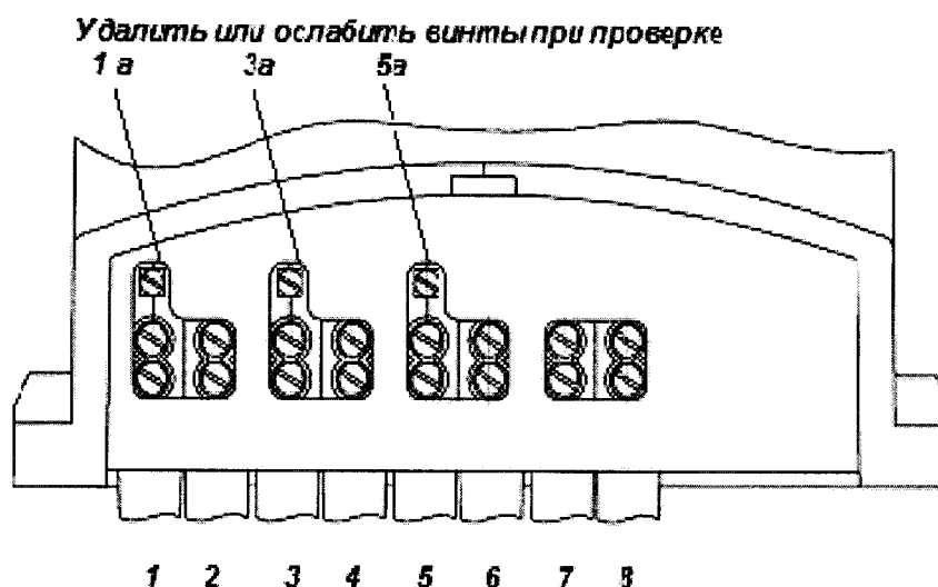
Рисунок Г.2 - Схема расположения контактов счетчиков РиМ 489.2Х на клеммной колодке
