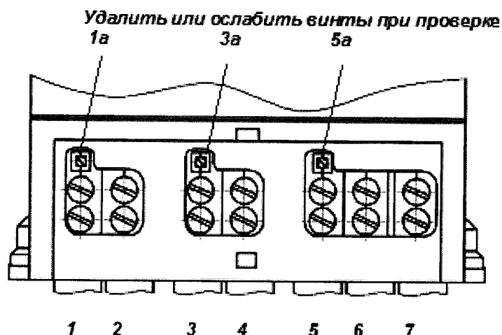
Рисунок Г.1 – Схема расположения контактов счетчиков РиМ 489.1Х на клеммной колодке
