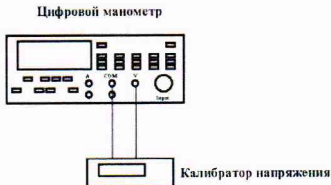
Рисунок 4. Схема поверки канала измерений напряжения постоянного электрического тока.
