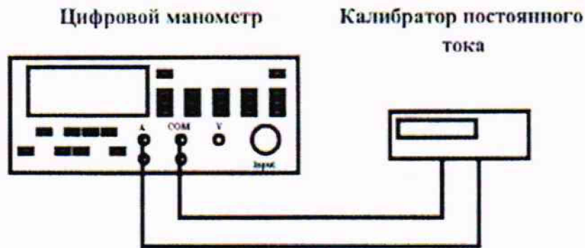
Рисунок 3. Схема поверки канала измерений силы постоянного электрического тока.
