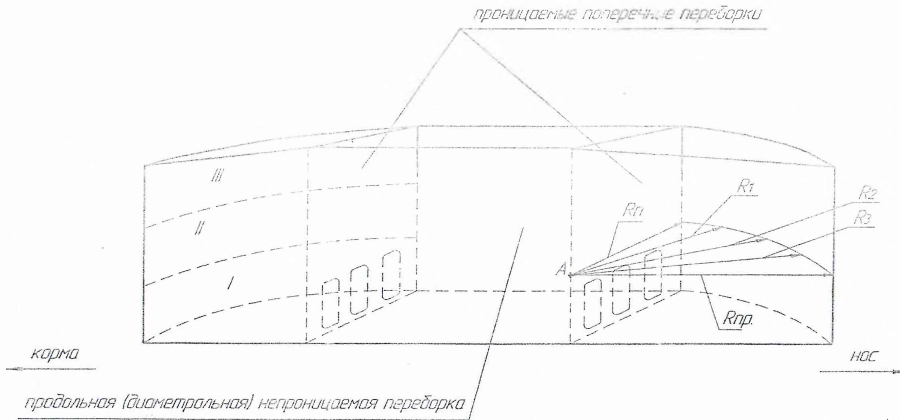
Рисунок А.7 – Схема измерений параметров цилиндрической части
