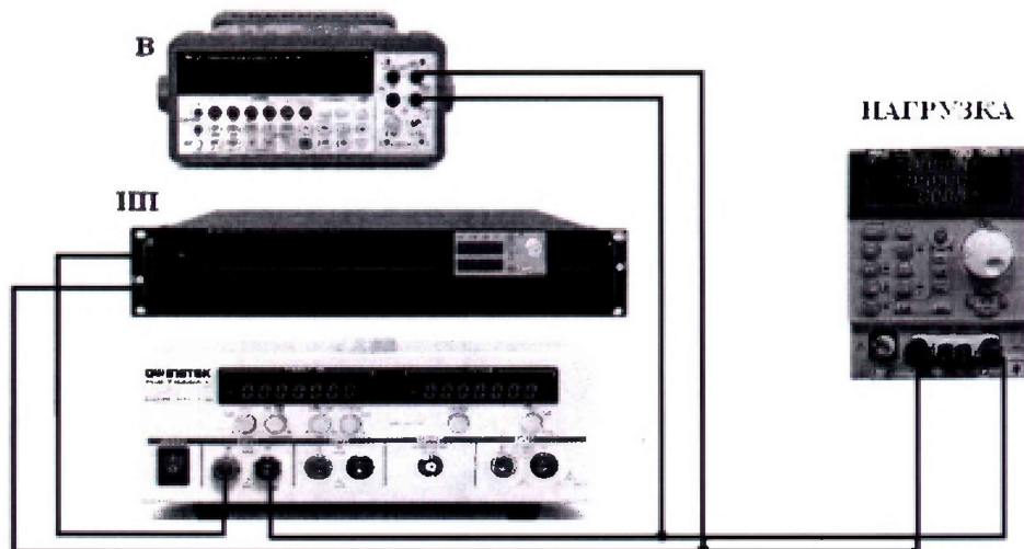
Рисунок 3 - Схема подключения приборов при определении абсолютной погрешности установки и измерений мощности при работе в режиме стабилизации мощности постоянного тока.
