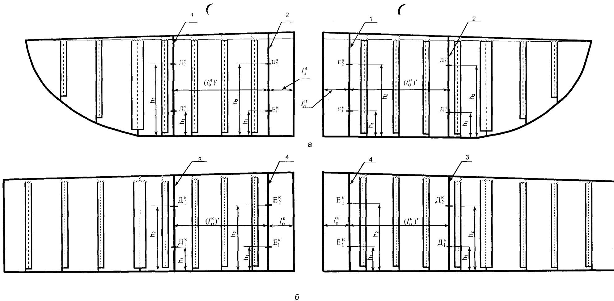
а – носовая поперечная переборка левого и правого бортов; б – кормовая поперечная переборка левого и правого бортов; 1,2,3,4 – вертикальные линии; D_1^H, D_1^K, E_1^H, E_1^K, D_2^H, D_2^K, E_2^H, E_2^K – точки на вертикальных линиях; l_0^H, l_0^K – расстояния от продольной переборки до линий 1 и 4; (l_0^H)', (l_0^K)' – расстояния между линиями 1,2 и 3,4; h_1 – высота точек D_1 и E_1 ; h_2 – высота D_2 и E_2 .
