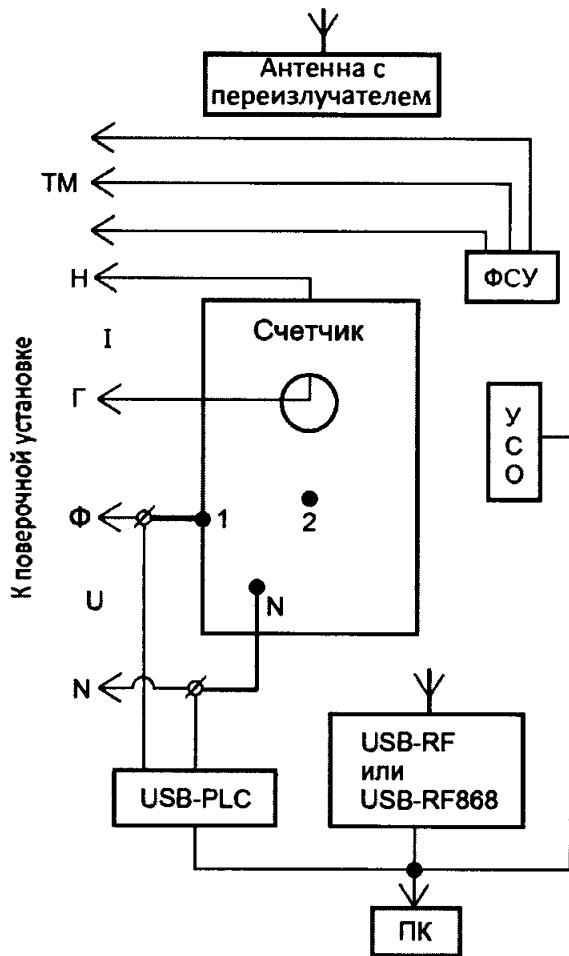
Рисунок Б.1 – Схемы включения счетчиков в корпусе «тип I»
