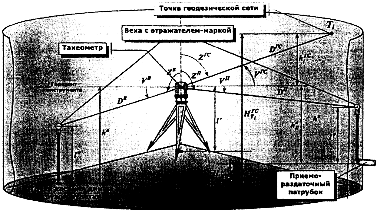
Рисунок А.3 Определение абсолютной высоты точки геодезической сети и „мертвой” полости относительно точки касания дна груза рулетки при установке тахеометра внутри резервуара
