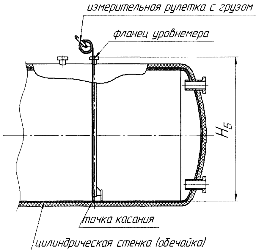
Рисунок А.2 – Схема измерений базовой высоты
