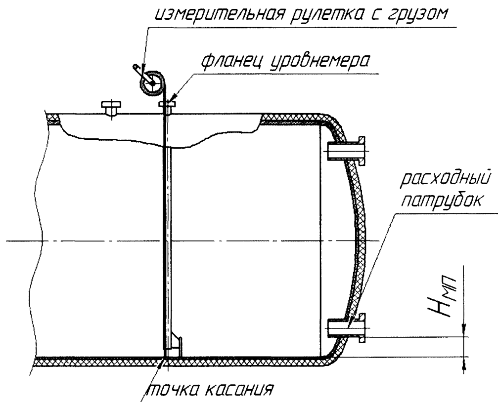
Рисунок А.4 – Схема измерений высоты мертвой полости
