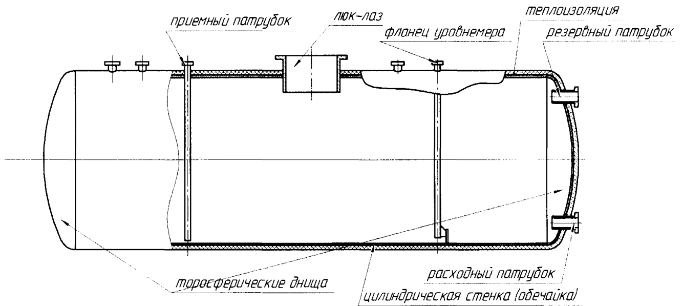
Рисунок А.1 – Общий вид резервуара РГС-100
